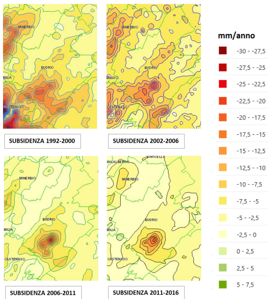
Figura 15 - Isocinetiche 1992-2015
